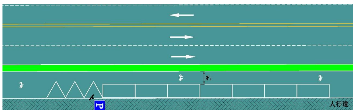
图2 设置停车位后非机动车专用道剩余宽度示例
