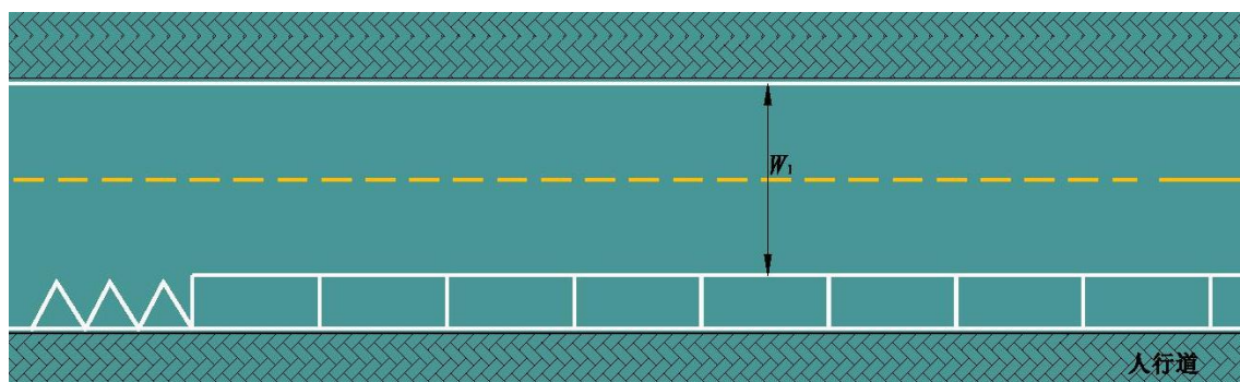
图1 设置停车位后车行道剩余宽度示例
