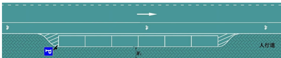
图3 占用人行道设置港湾式停车位后人行道剩余宽度示例
